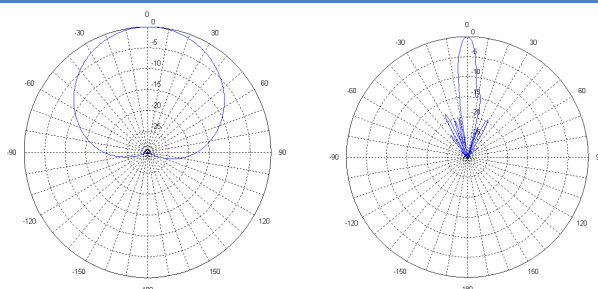
2GHz方向图
