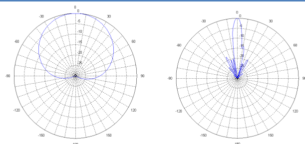
800M方向图
