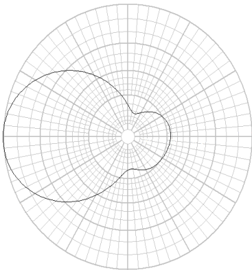
垂直面方向图
