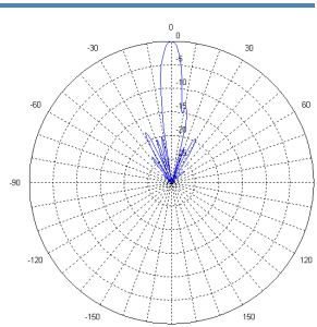
820-960/1710-2170MHz
